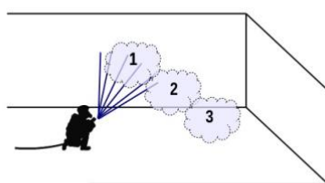
Fig 19. Pulsaciones para el control de gases o la extinción de llamas.
