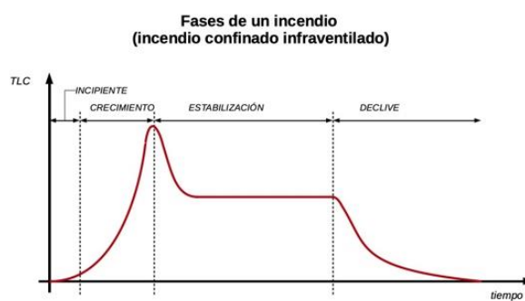
Fig 11. Ejemplo de un posible desarrollo de incendio en el que el recinto ejerce una influencia importante sobre el incendio: la potencia del mismo está limitada por la capacidad de intercambio de gases. En la gráfica se identifican las fases típicas.
